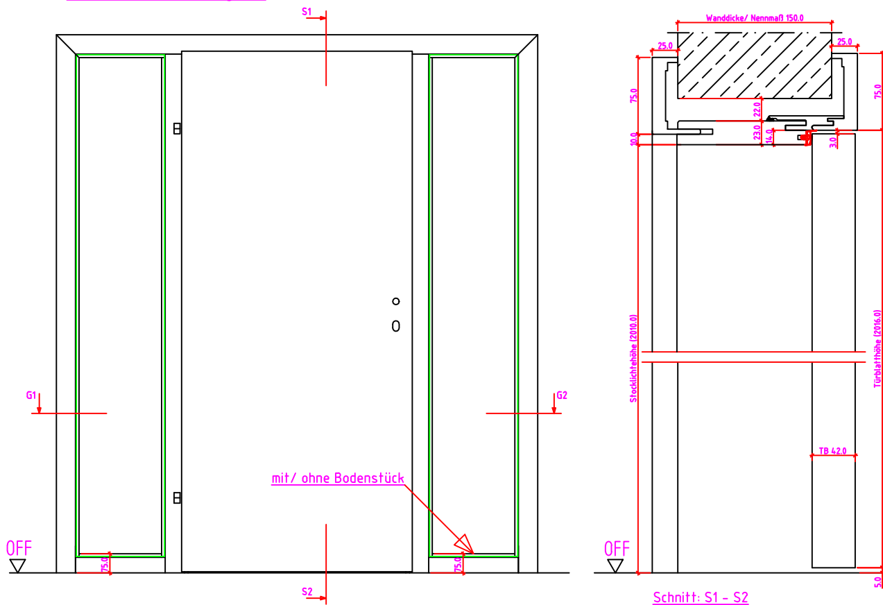
Ansicht: WF-Z 2S Anschlag links
