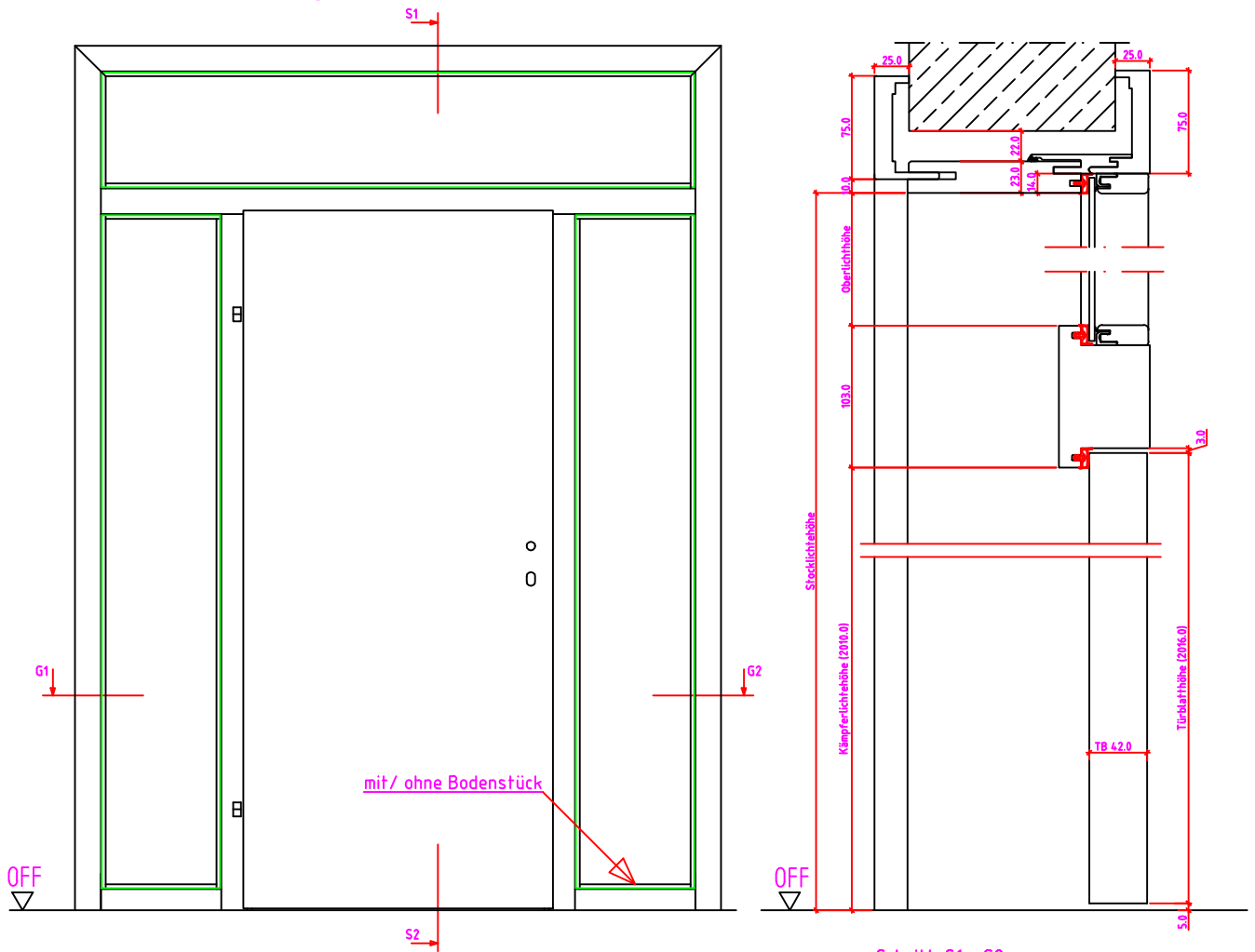
Ansicht: WF-Z 2SK Anschlag links
