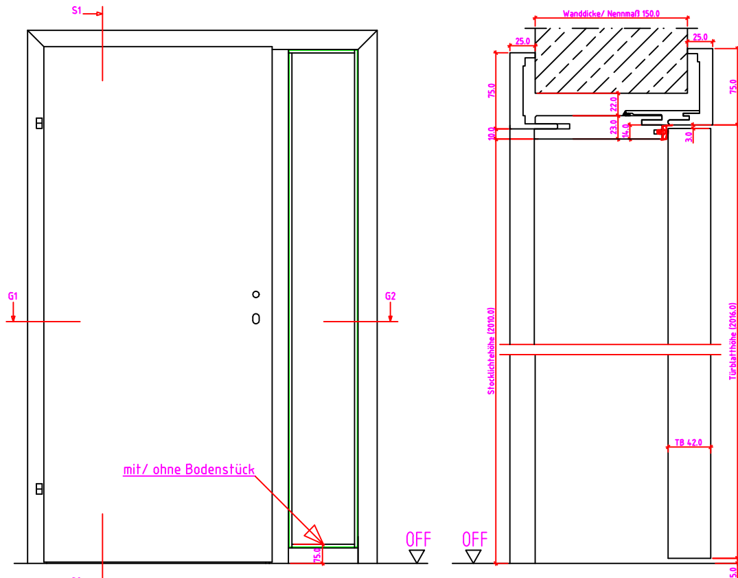
Schnitt: S1 - S2
