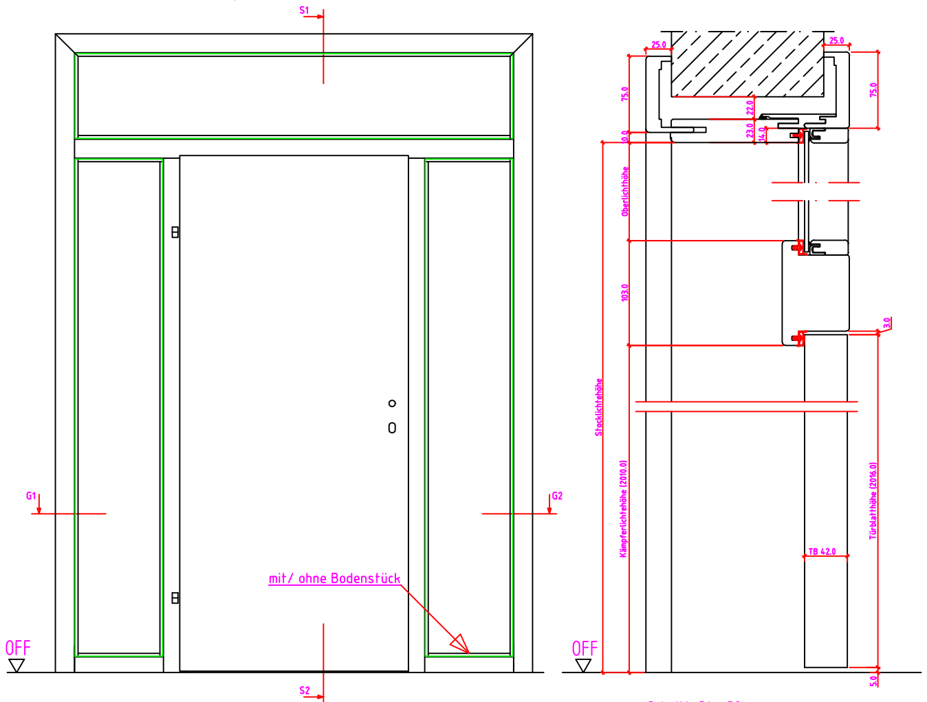
Schnitt: S1 - S2
