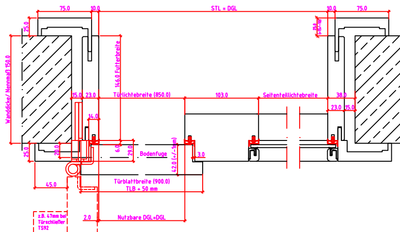
Grundriss: G1 - G2
