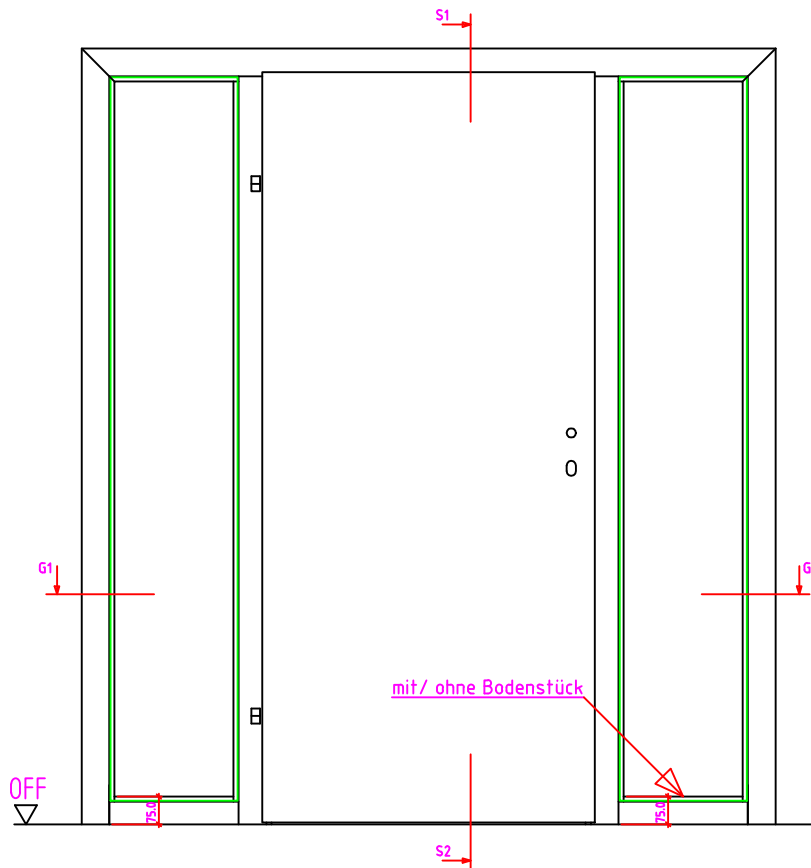
Ansicht: WF-Z 2S Anschlag links
