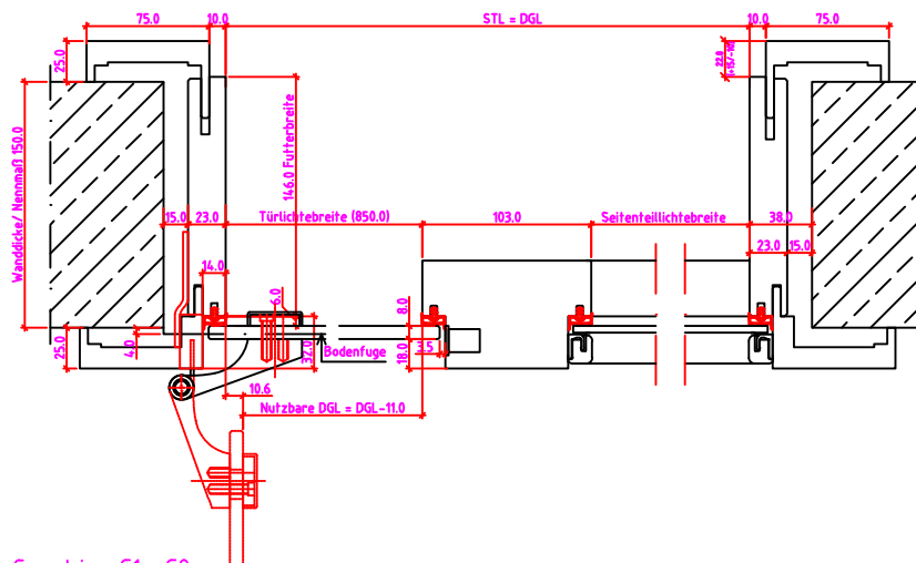
Grundriss: G1 - G2
