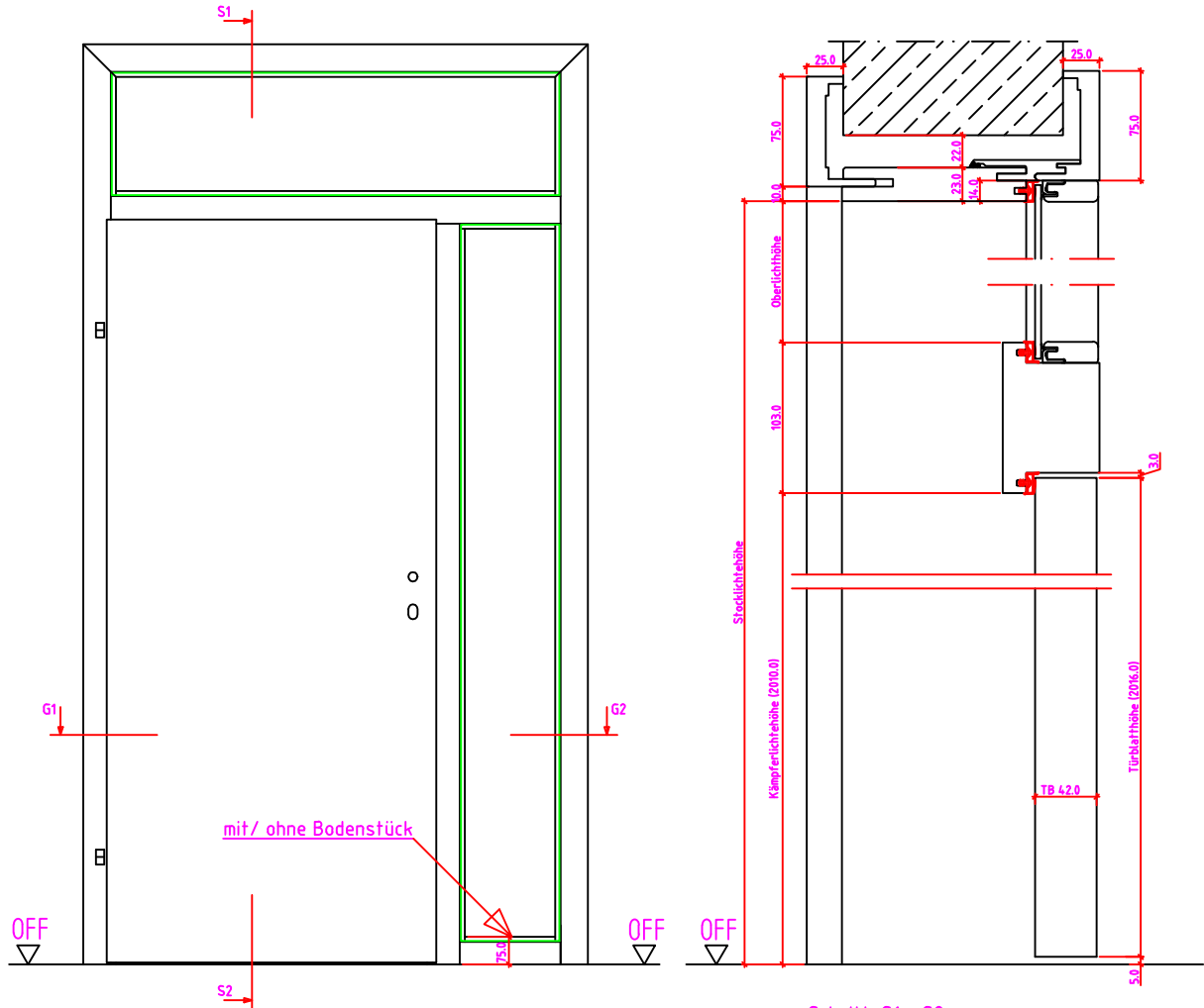
Schnitt: S1 - S2
