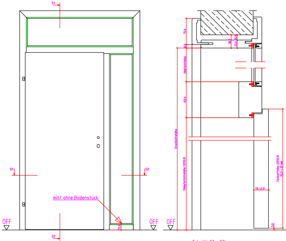
Ansicht: WF-Z 1SK-R Anschlag links
