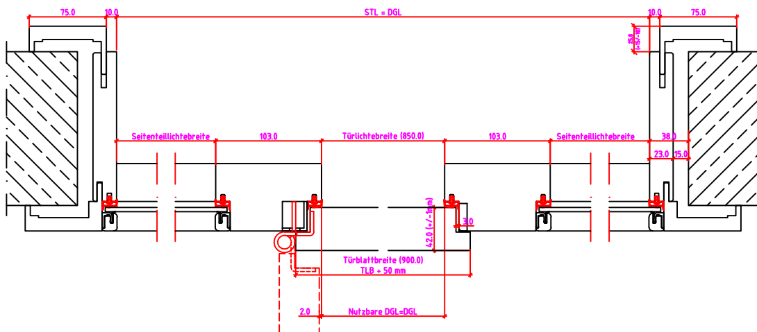
Grundriss: G1 - G2
