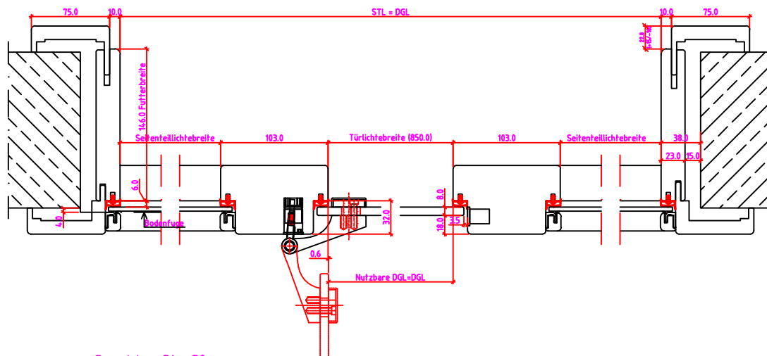
Grundriss: G1 - G2
