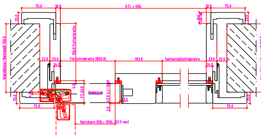
Grundriss: G1 - G2
