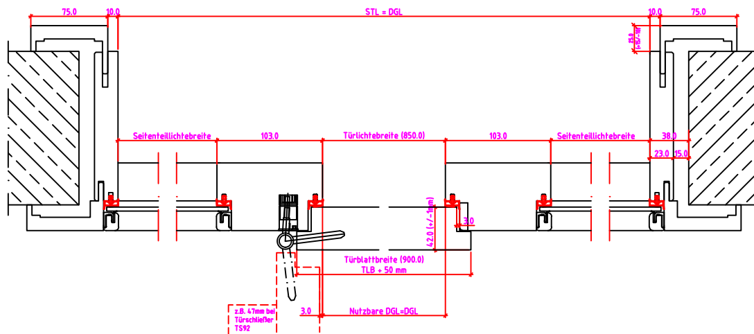
Grundriss: G1 - G2
