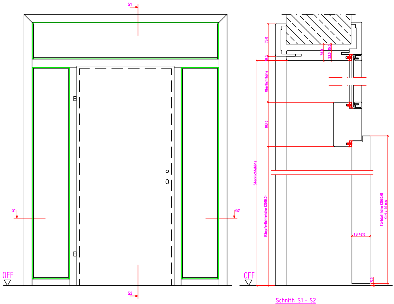
Ansicht: WF-Z 2SK Anschlag links
