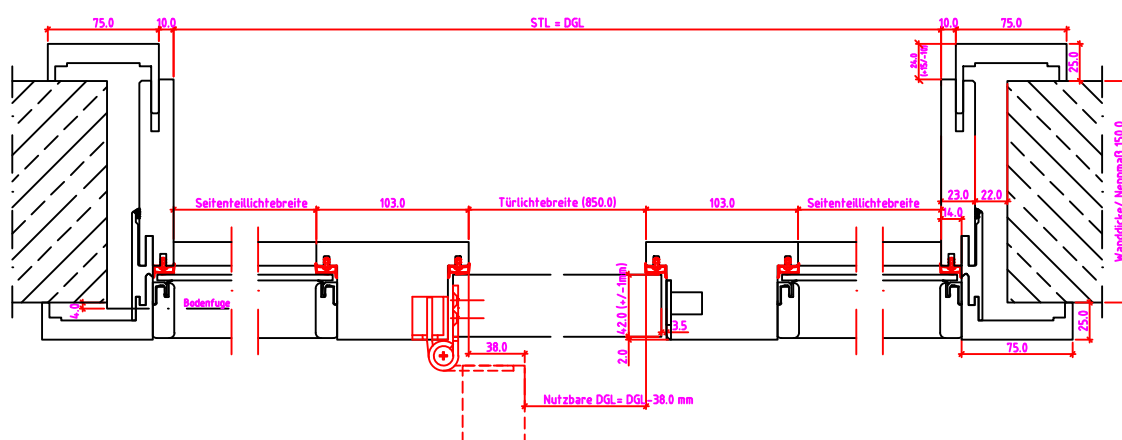
Grundriss: G1 - G2
