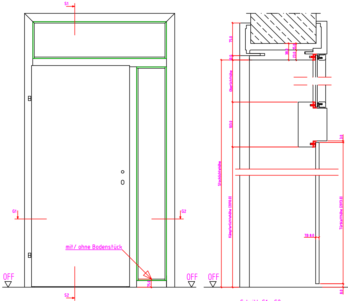
Ansicht: WF-Z 1SK-R Anschlag links
