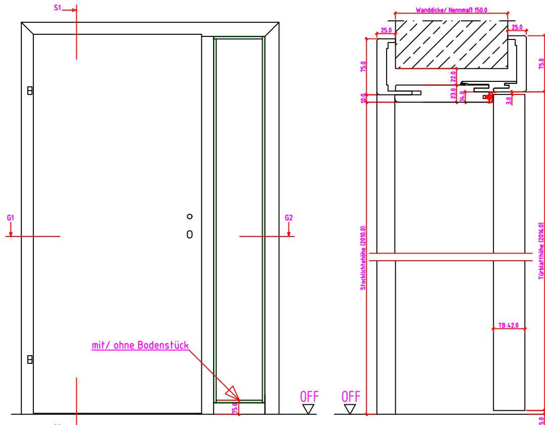
Ansicht: WF-Z 1S-R Anschlag links
