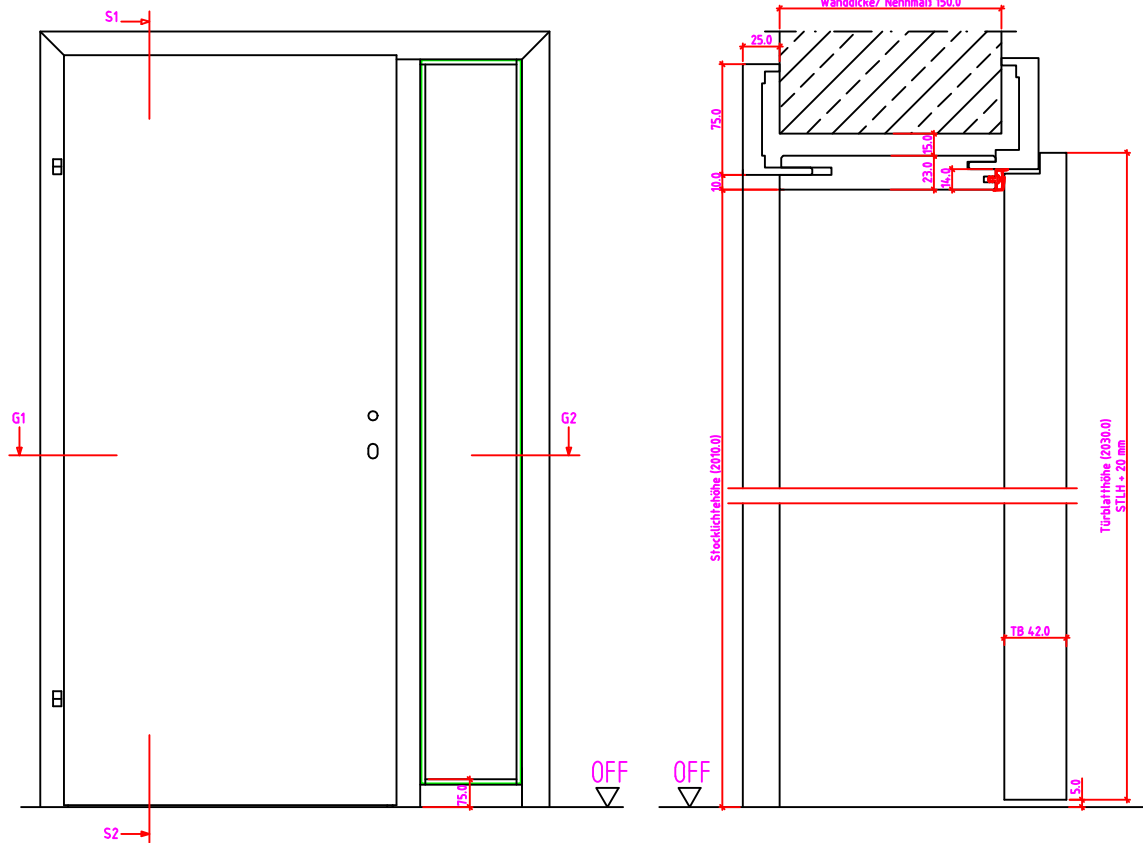
Schnitt: S1 - S2
