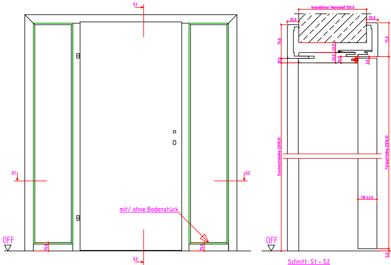
Ansicht: WF-Z 2S Anschlag links
