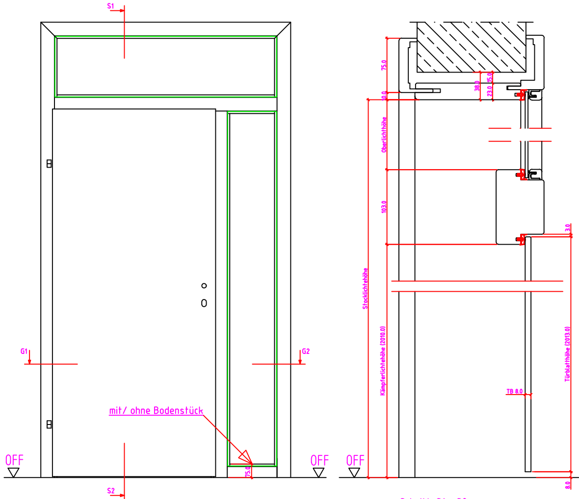
Schnitt: S1 - S2
