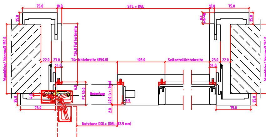
Grundriss: G1 - G2
