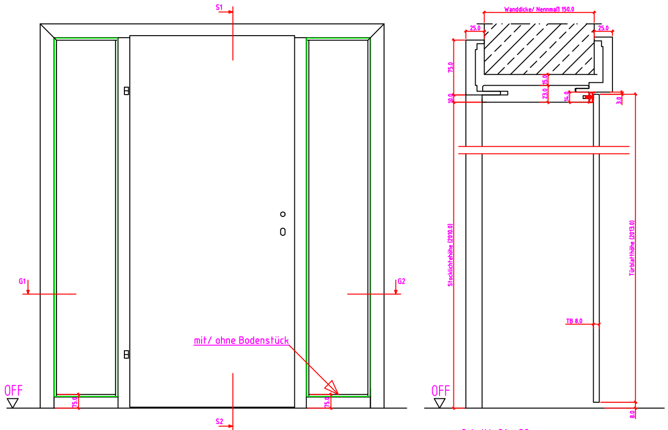
Schnitt: S1 - S2
