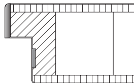
Starkfurnier-, ABS- oder Kompaktkante mit Furnier- oder Kunststoffkante, Brandschutzquellstreifen sichtbar
