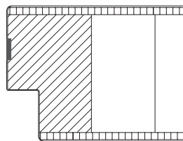
Furnier- oder Kunststoffkante Brandschutzquellstreifen sichtbar
