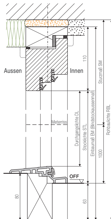
Schnitt K1 - K2
