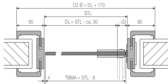
Schnitt G3 - G4 Ganzglas Türblatt (GT):
