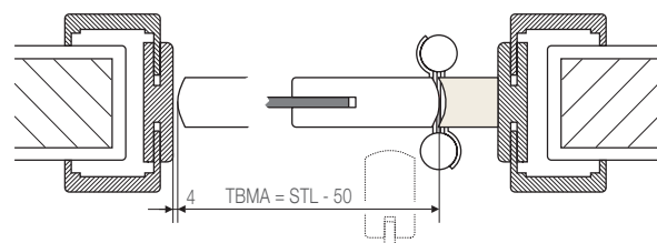
Schnitt G7 - G8 Friesglas Türblatt (FG):
