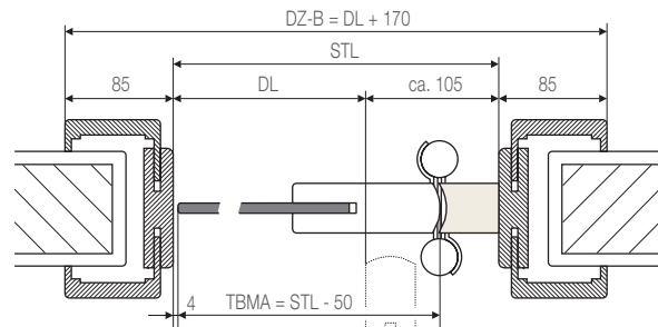
Schnitt G5 - G6 Halbglass Türblatt (HG):
