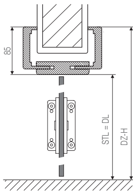
Schnitt K3 - K4 Ganzglas Türblatt (GT):
