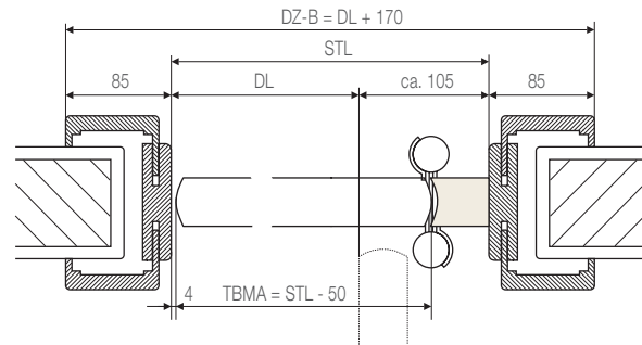
Schnitt G3 - G4 Ganzglas Türblatt (GT):
