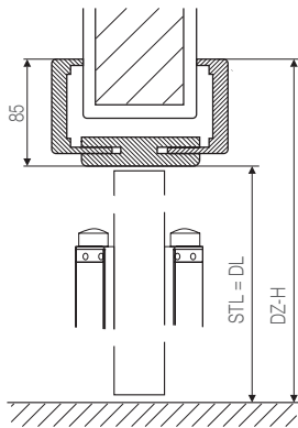
Schnitt K1 - K2 Standard Türblatt:
