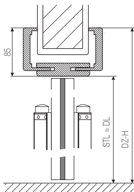
Schnitt K5 - K6 Halbglass Türblatt (HG): Friesglas Türblatt (FG):
