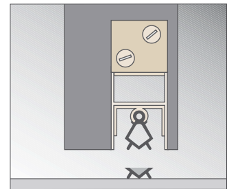
Absenktdichtung
