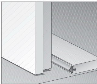
Türstapel (Schwelle) mit Dichtung
