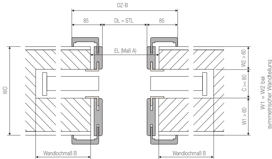
Schnitt G1 - G2
