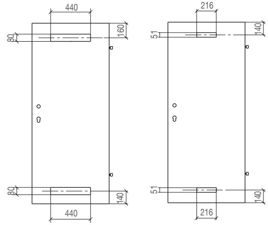
Fräsungen für Luftschlitze
