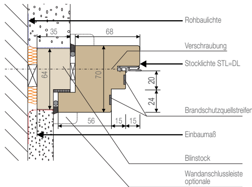
Schnitt G1 - G2 (M 1:4)
