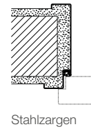
Stahlzargen
