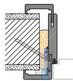
F97m/EI30 Modul
